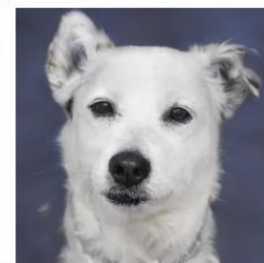
LLaMA-65B
