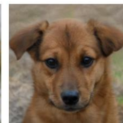
Bloom-7B
