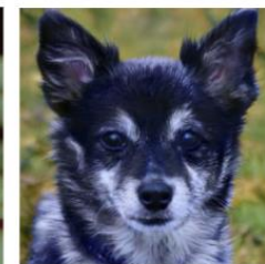
Galactica-120B
