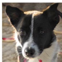
Pythia-12B
