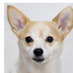
GPT-NeoX-20B
