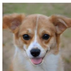
LLaMA2-13B
