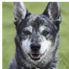
LLaMA-30B
