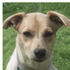
ChatGLM-6B
