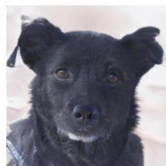
LLaMA-7B
