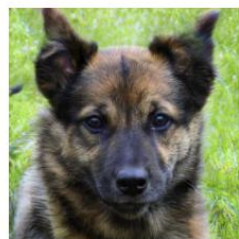
ChatGLM2-6B
