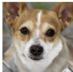
OPT-30B
