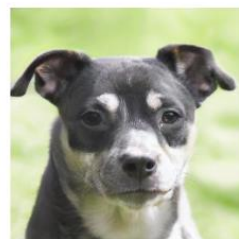
OpenLLaMA-7B
